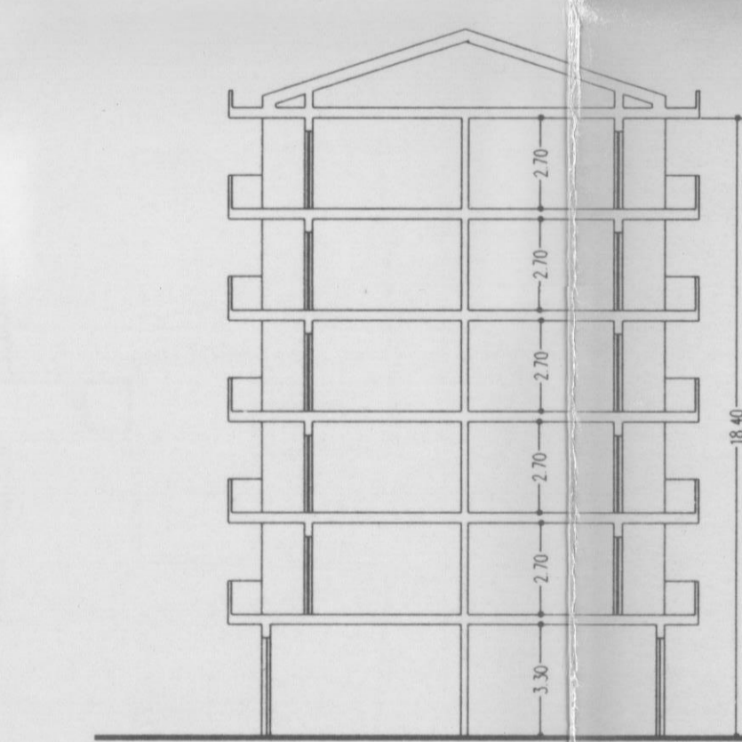
SEZIONE A-A
