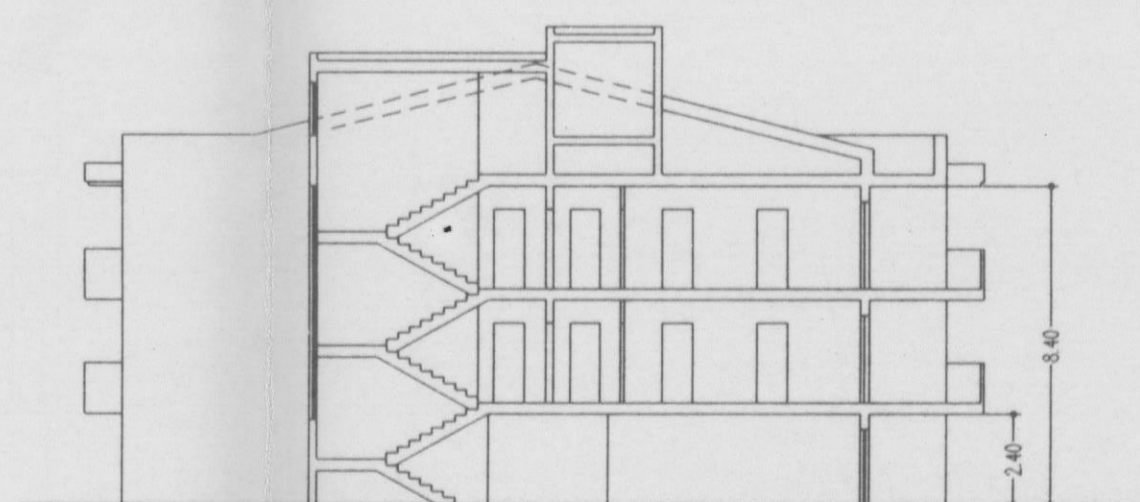
SEZIONE A-A
