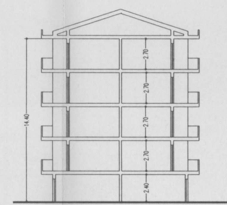
SEZIONE A-A
