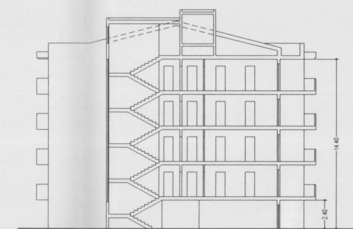
SEZIONE A-A
